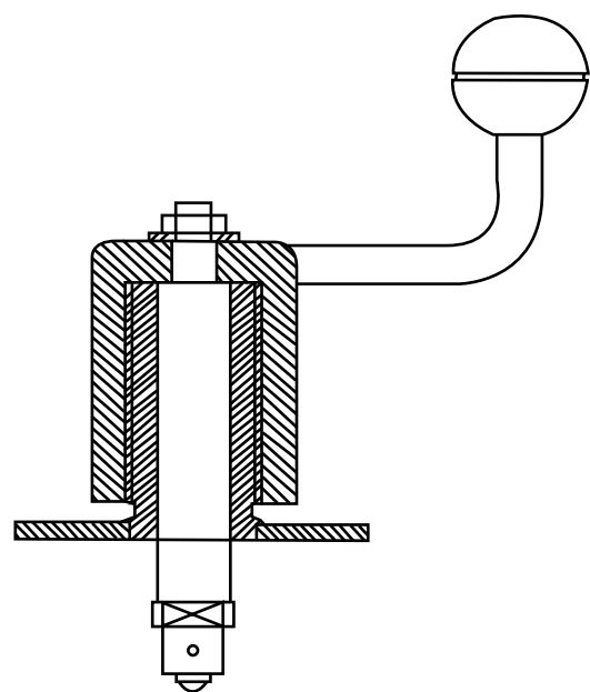
Manual Actuator
